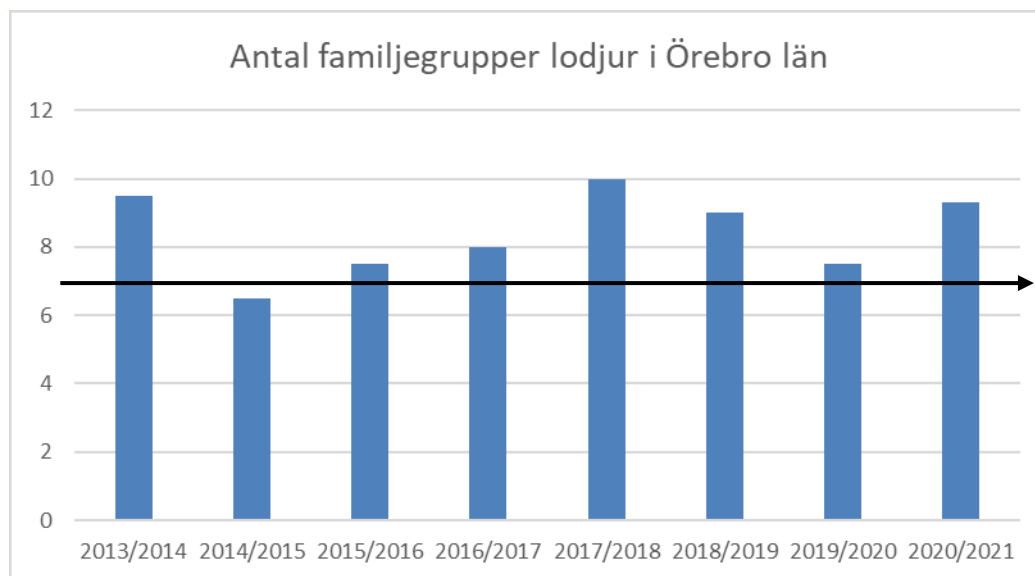
Figur 2: Inventeringsresultat i Örebro län inventeringssäsongerna 2013/2014 till 2020/2021. Länets aktuella miniminivå är av Naturvårdsverket beslutad till sju familjegrupper, visas som en svart pil i diagrammet. Innan inventeringssäsongen 2018/2019 var Örebro läns miniminivå beslutad av Naturvårdsverket till 9,5 familjegrupper.
