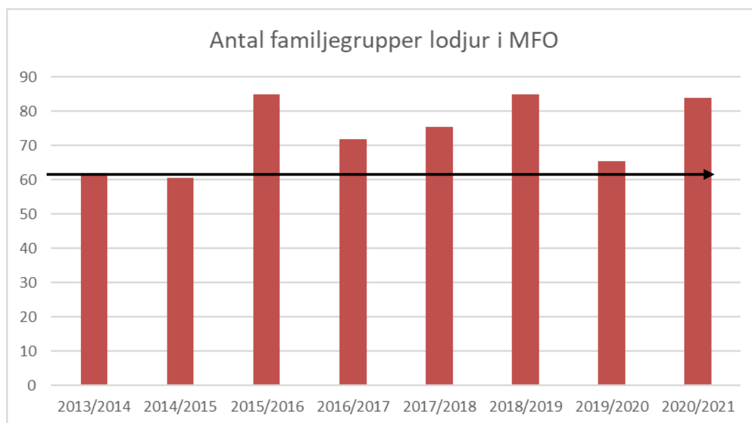
Figur 1: Inventeringsresultat i mellersta förvaltningsområdet inventeringsåren 2013/2014 till 2020/2021. Förvaltningsområdets miniminivå är av Naturvårdsverket beslutad till 62 föryngringar per år, miniminivån visas med en svart genomgående pil i figuren.
