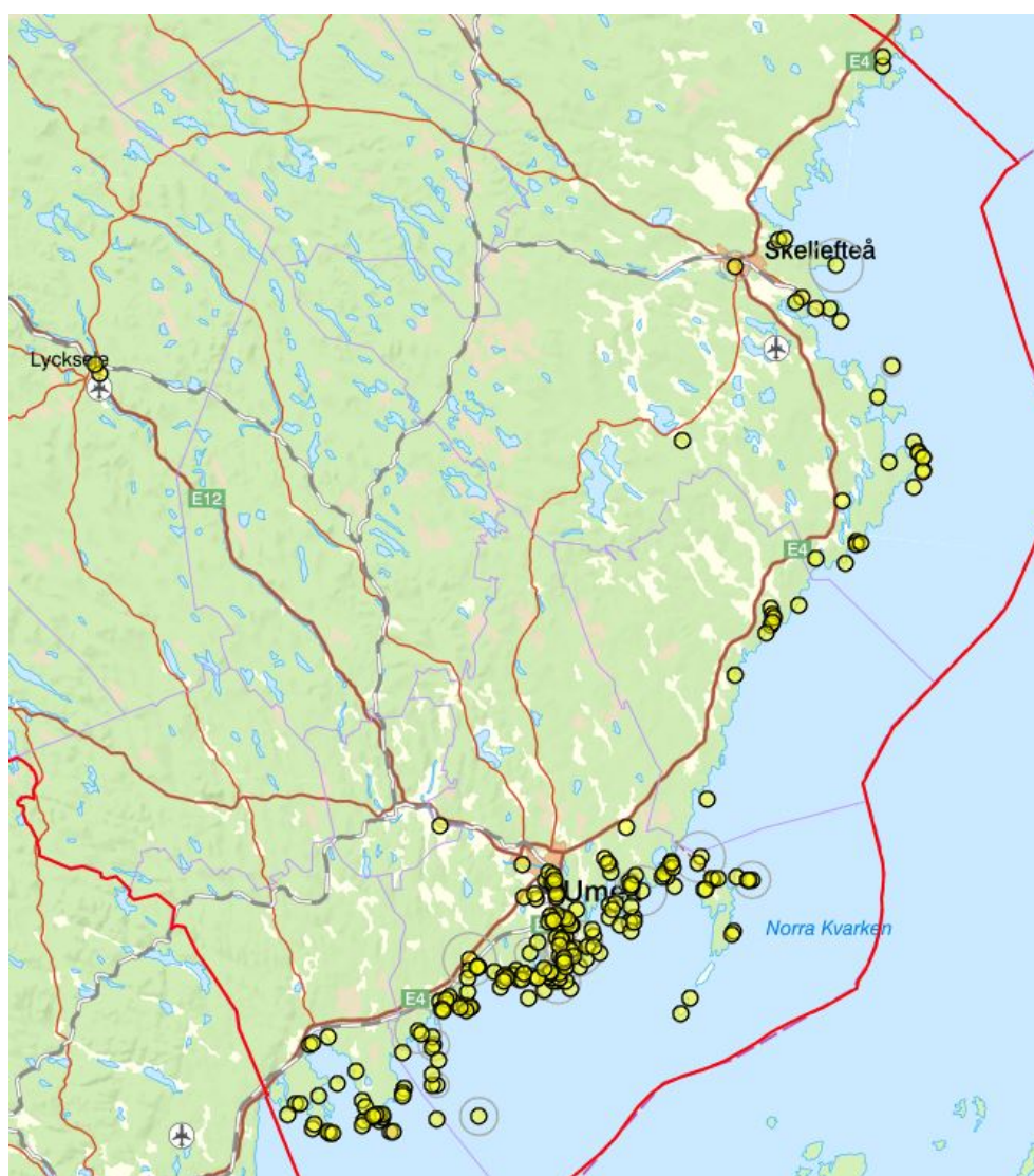
Figur 1: Observationer av skarv i Västerbotten under 2020-2021.
