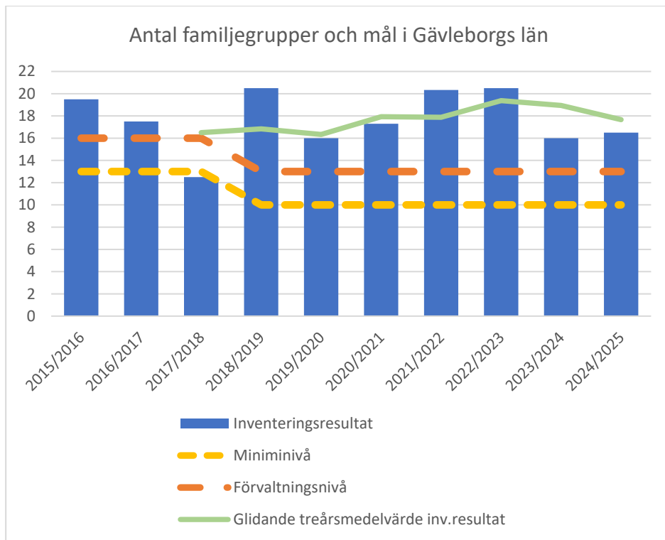
Figur 2 Resultatet av lodjursinventeringen i Gävleborgs län under perioden 2014/2015 till 2023/2024, glidande treårsmedelvärden av inventeringsresultatet samt gällande miniminivå och förvaltningsnivå.
