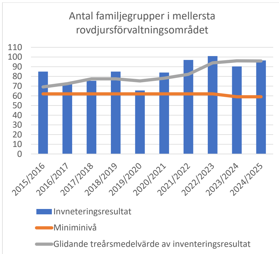
Figur 1. Inventeringsresultat, glidande treårsmedelvärde av inventeringsresultat samt gemensam miniminivå i mellersta rovdjursförvaltningsområdet åren 2015/2016–2024/2025
