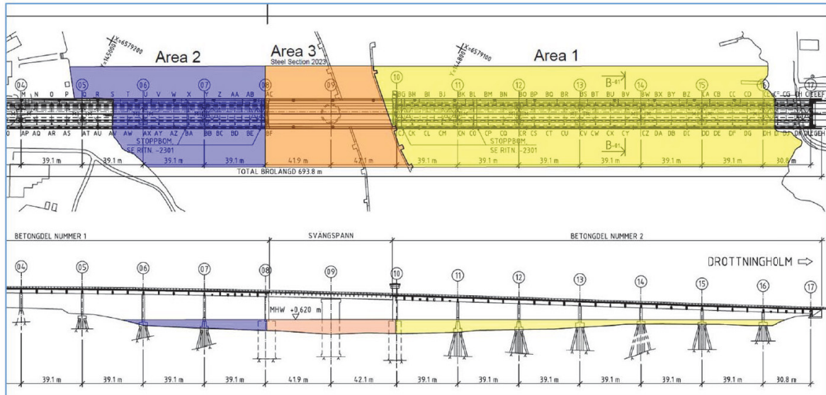
Figur 1. Indelning av brospannen på Nockebybron.
