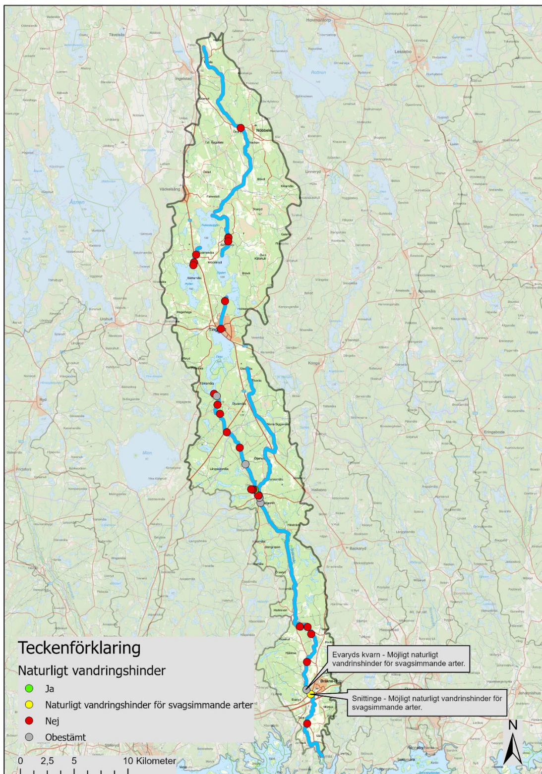
Figur 1. Karta som visar artificiella vandringshinder och om de anses vara naturliga eller inte i Bräkneåns provningsområde. Datan är inhämtad från biotopkarteringsdatabasen 2022-10-31 och från Länsstyrelsen Kronoberg. Snittinge och Evaryds kvarn är artificiella vandringshinder som är belägna vid naturliga vandringshinder. Evaryds kvarn och Snittinge är passerbara för starksimmande arter i referensförhållandet men möjligen partiellt eller definitivt för svagsimmande arter. Placeringen preciseras i kartan.
