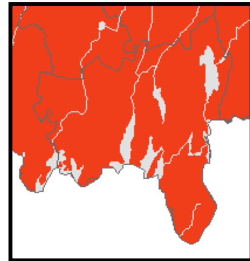
Beräknat 2069-2098
