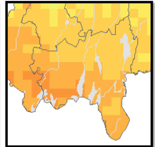
Beräknat 2069-2098
