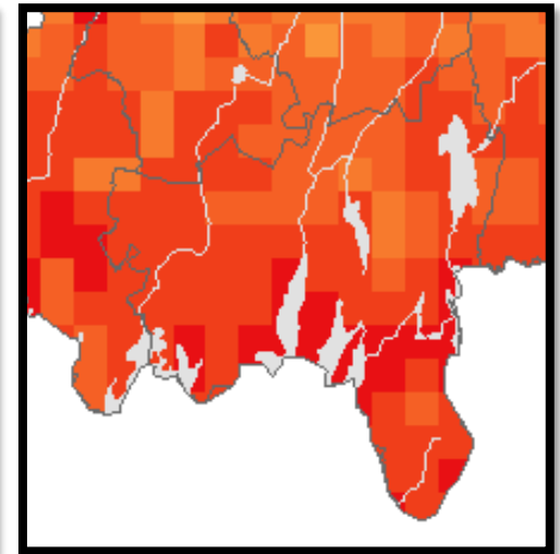
Beräknat 2069-2098
