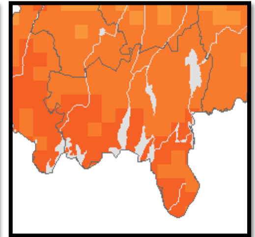
Beräknat 2069-2098
