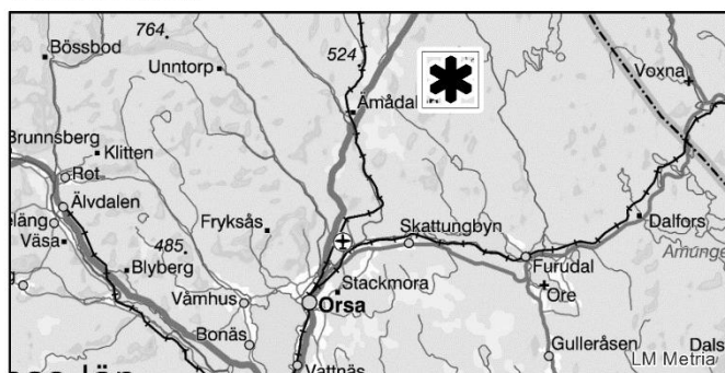
Översigtskarta
