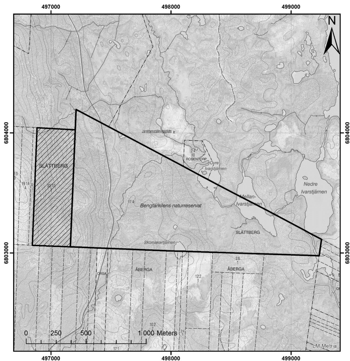
Översigtskarta
