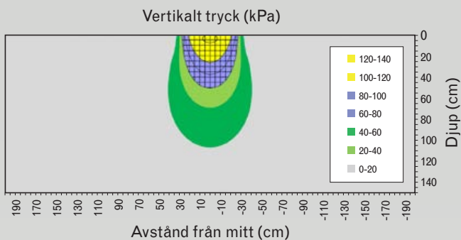
Tryckutbredning i jordprofilen för enkelmontage med ca 3 500 kg hjullast och 0,8 bar.
