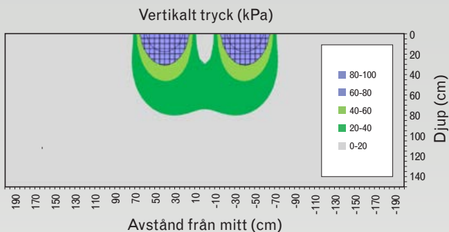
Tryckutbredning i jordprofilen för dubbelmontage monterad på samma traktor (halverad hjullast och därmed behov av lägre ringtryck, 0,6 bar)
