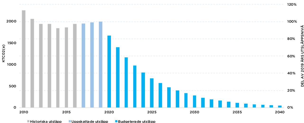
Figur 1. Historiska utsläpp 9 2010–2016, uppskattade utsläpp 2017–2019, samt budgeterade utsläpp 2020–2040. Utsläppen föreslås minska med en konstant andel av föregående års utsläpp. Den högra Y-axeln visar utsläpp som procent av basåret 2019.
