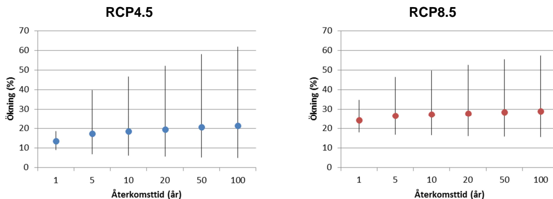
Figur 4. Procentuell förändring av nederbörd med varaktigheten 1 timme mellan perioderna 2069-2098 och 1961-1990 för Gotlands län. Punkterna representerar medianvärden och vertikala streck visar spridningen mellan de olika modellberäkningarna.
