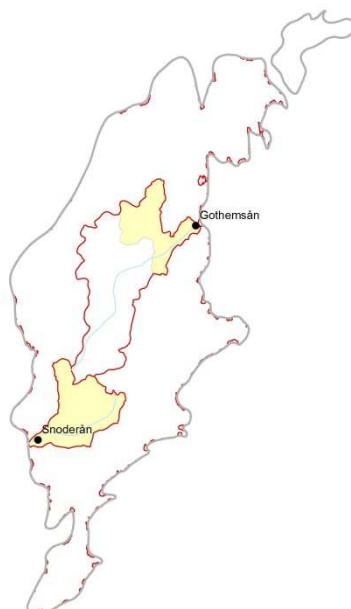
Figur 5. Kartan visar avrinningsområden (röda linjer) och de markerade vattendragspunkterna relaterar till diagrammen över total tillrinning i rapporten. De gulmarkerade områdena avser beräkningarna för lokal tillrinning och markfuktighet. Gotlands län markeras med grå linje.
